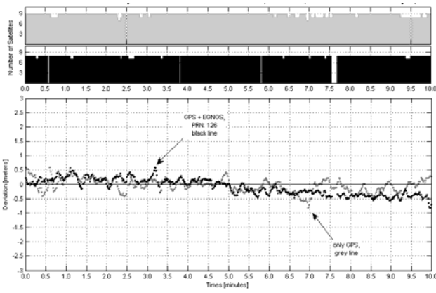
Fig. 7. Septentrio Y Coordinate Deviation, 0 Deg. Mask
