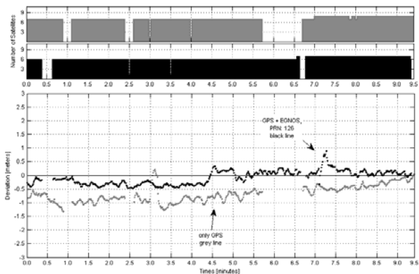
Fig. 2. Septentrio Y Coordinate Deviation, 15 Deg. Mask
