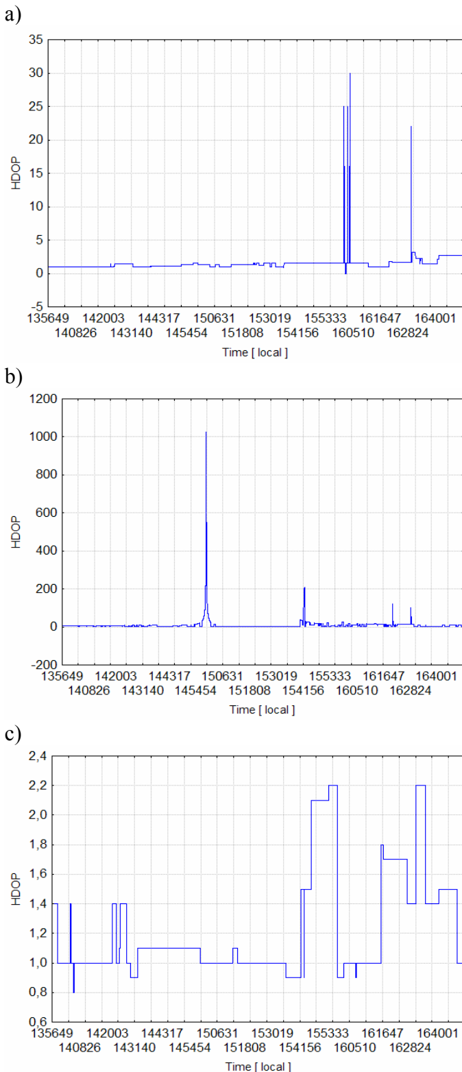
Fig. 4. HDOP factor in measuring points: a) Glinki, b) ul. Bolesława Śmiałego c) AM Szczecin (date: 2006-10-26)
